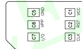
SIM 示意图 芯片面朝下视图
