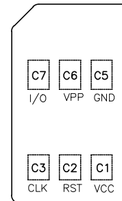
SIM 示意图 芯片面朝下视图
