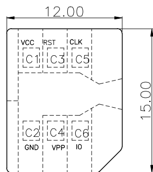
芯片面朝下视图
