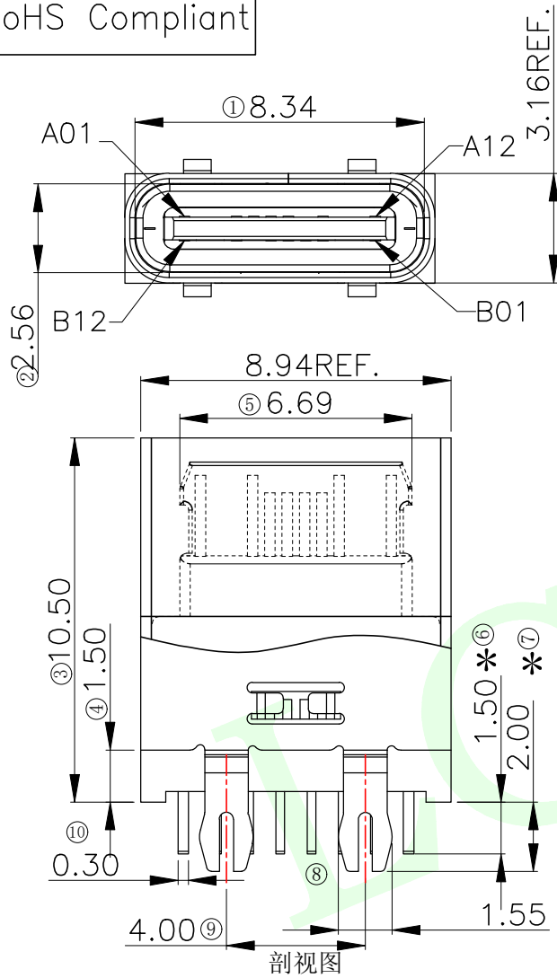
剖视图
