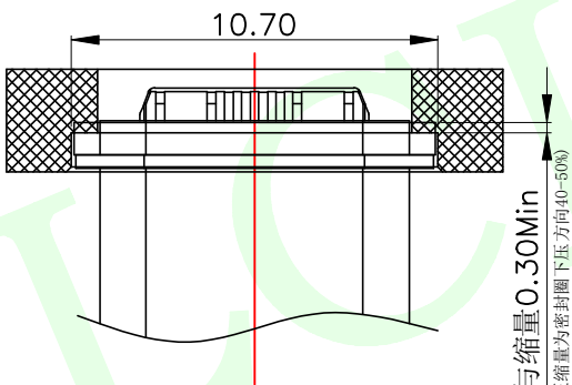
直压结构密封参考尺寸
