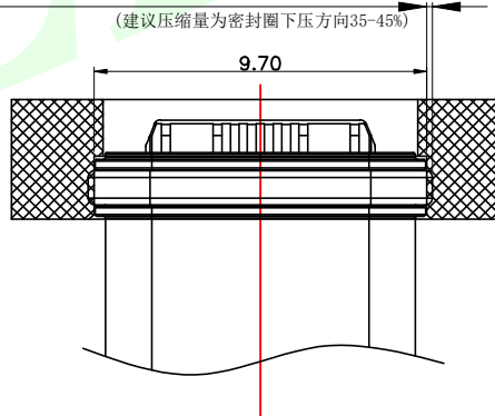
U型结构密封参考尺寸
