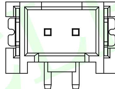
2 PIN 结构样式 (Structural style)
