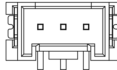
3 PIN 结构样式 (Structural style)
