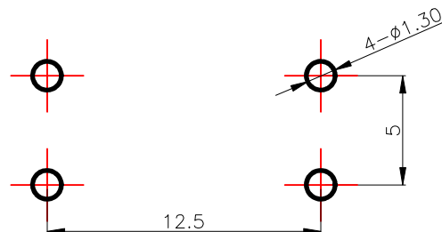
PCB. 焊接图
