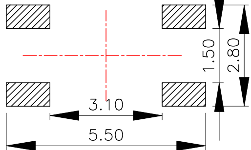
PCB. 焊接图
