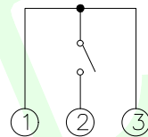
电路图
