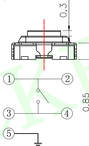
电路图
