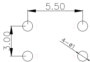
PCB. 焊接图
