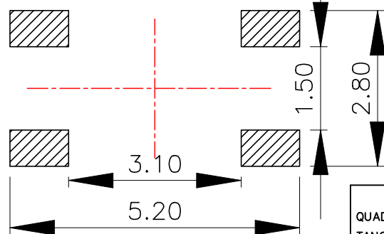
PCB. 焊接图
