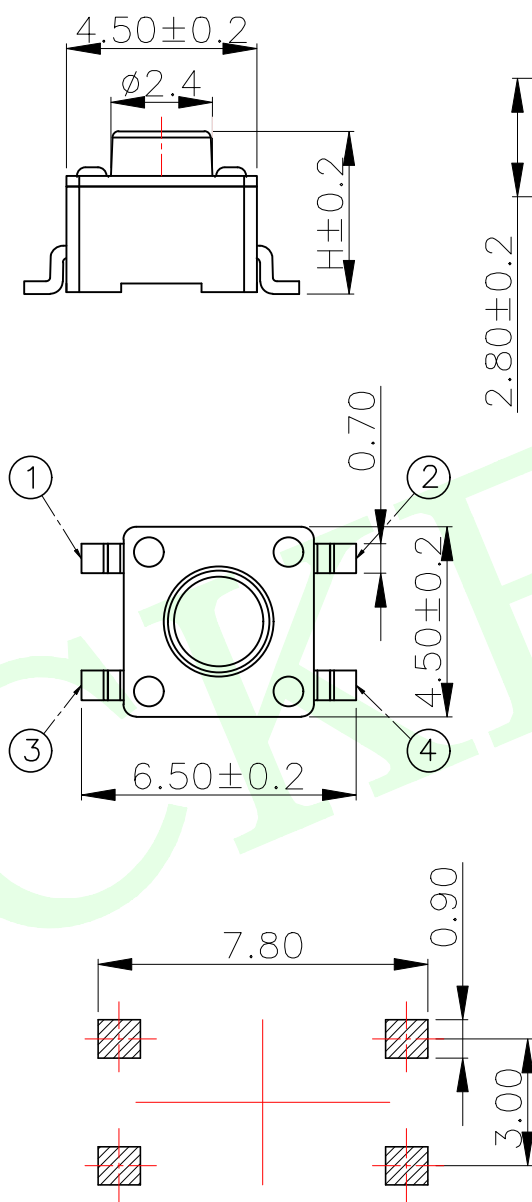
PCB. 焊接图
