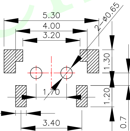
PCB. 焊接图
