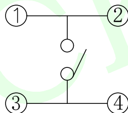
电路图
