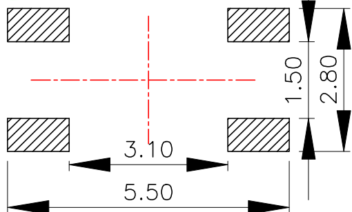
PCB. 焊接图
