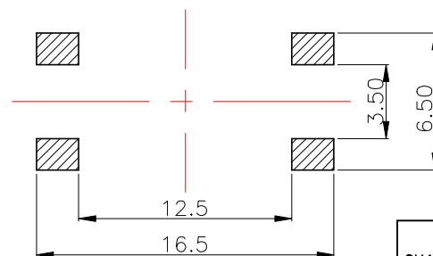
PCB. 焊接图
