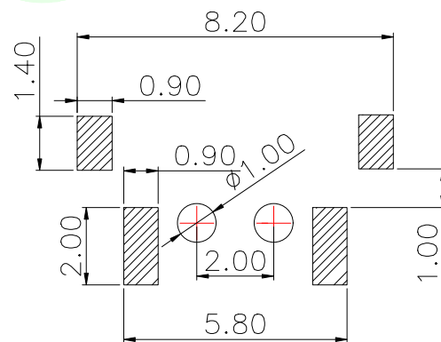
PCB. 焊接图
