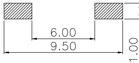
PCB. 焊接图
