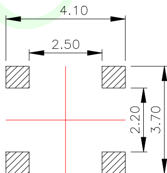
PCB. 焊接图
