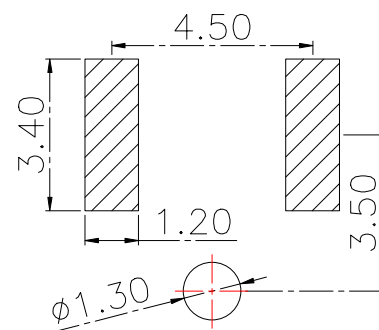
PCB. 焊接图
