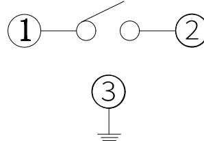
电路图
