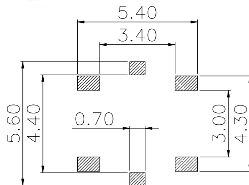
PCB. 焊接图
