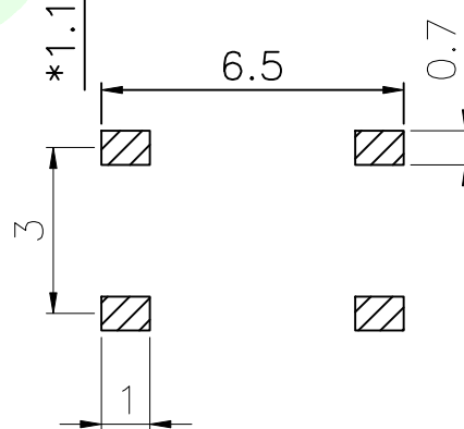
PCB. 焊接图
